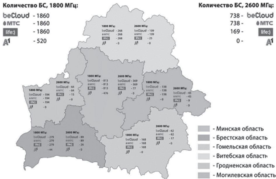
Рис. 1. Схема размещения базовых станций 4G — покрытия Беларуси (источник: URL: https://becloud.by/media-center/news/becloud-vypustil-novuyu-versiyu-onlayn-karty-4g-pokrytiya-belarusi/ (дата обращения: 01.02.2025))
